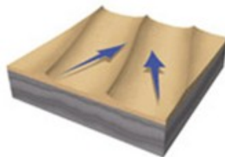
longitudinal dunes
